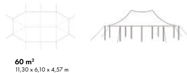
MODÈLE DE LARGEUR 6,10 M 6.10 M WIDE MODEL
